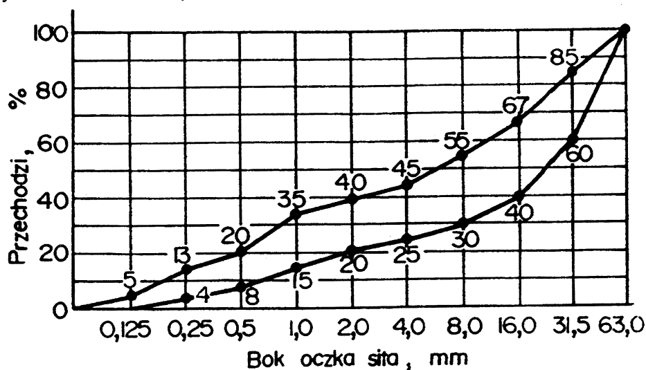
Rysunek 2. Graniczne krzywe uziarnienia kruszywa do betonu C 16/20 od 0 do 63 mm.
