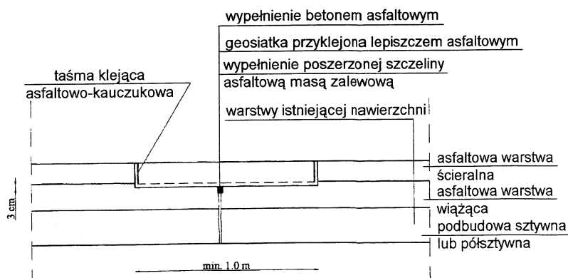
Rys. 1. Naprawa płytka pojedynczego pęknięcia odbitego, gdy krawędzie pęknięcia są dobrze podparte - w istniejącej warstwie ścieralnej
